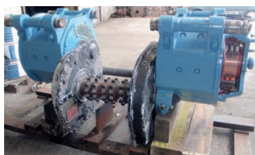
Réducteur de locotracteur Moyses CN 60 Gearmotor of a locomotive Moyses CN 60
